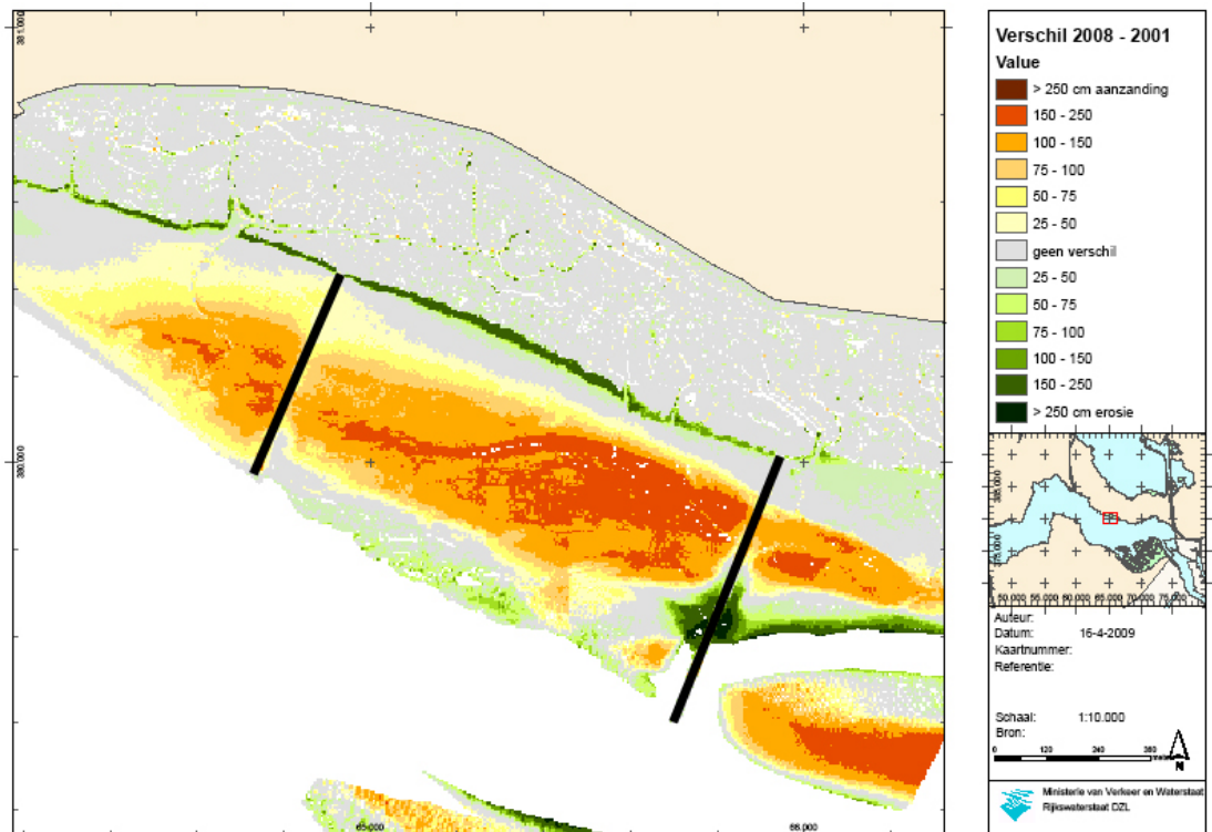
Schor van Waarde hoogteverschilkaart (oranje = opslibbing, groen = erosie)
