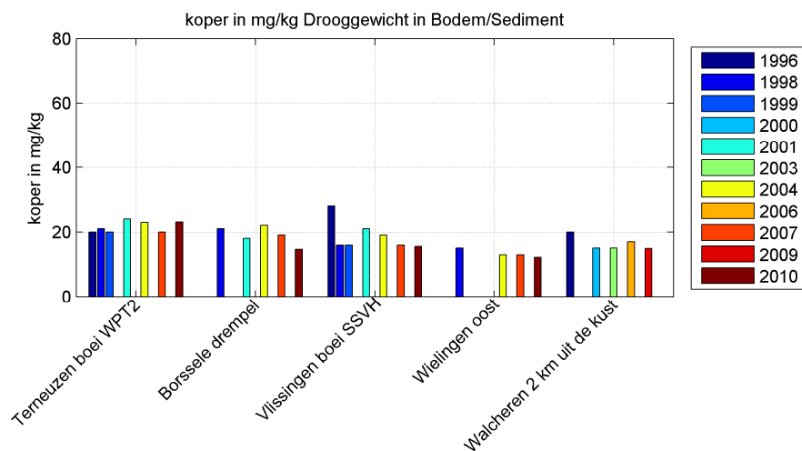
Figuur 3.95 Gemeten gehalten van koper in bodemsediment van de Westerschelde.
