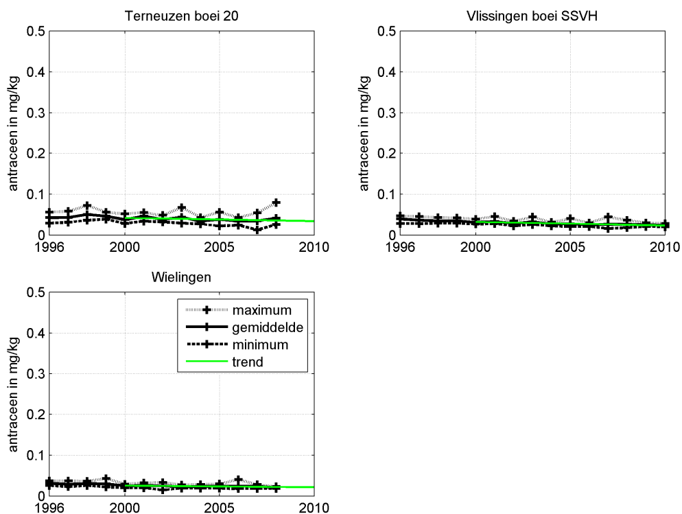
Figuur 3.77 Gemiddelde, minimum- en maximumwaarde per jaar van het gehalte antracene in zwevende stof op verschillende stations in het estuarium.
