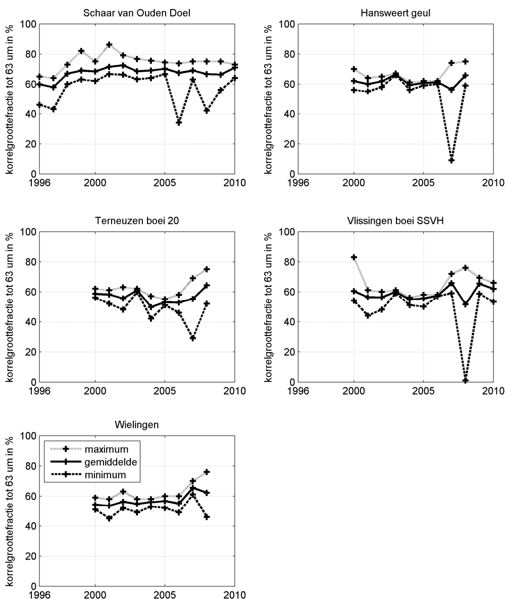
Figuur 3.59 Gemiddelde, minimum- en maximumwaarde per jaar van de fractie < 63 \mu\text{m} in zwevende stof op verschillende stations in het estuarium.
