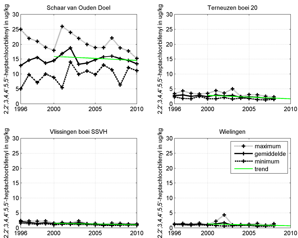
Figuur 3.70 Gemiddelde, minimum- en maximumwaarde per jaar van het gehalte 2,2',3,4,4',5,5'-heptachlorobifenyl in zwevende stof op verschillende stations in het estuarium.
