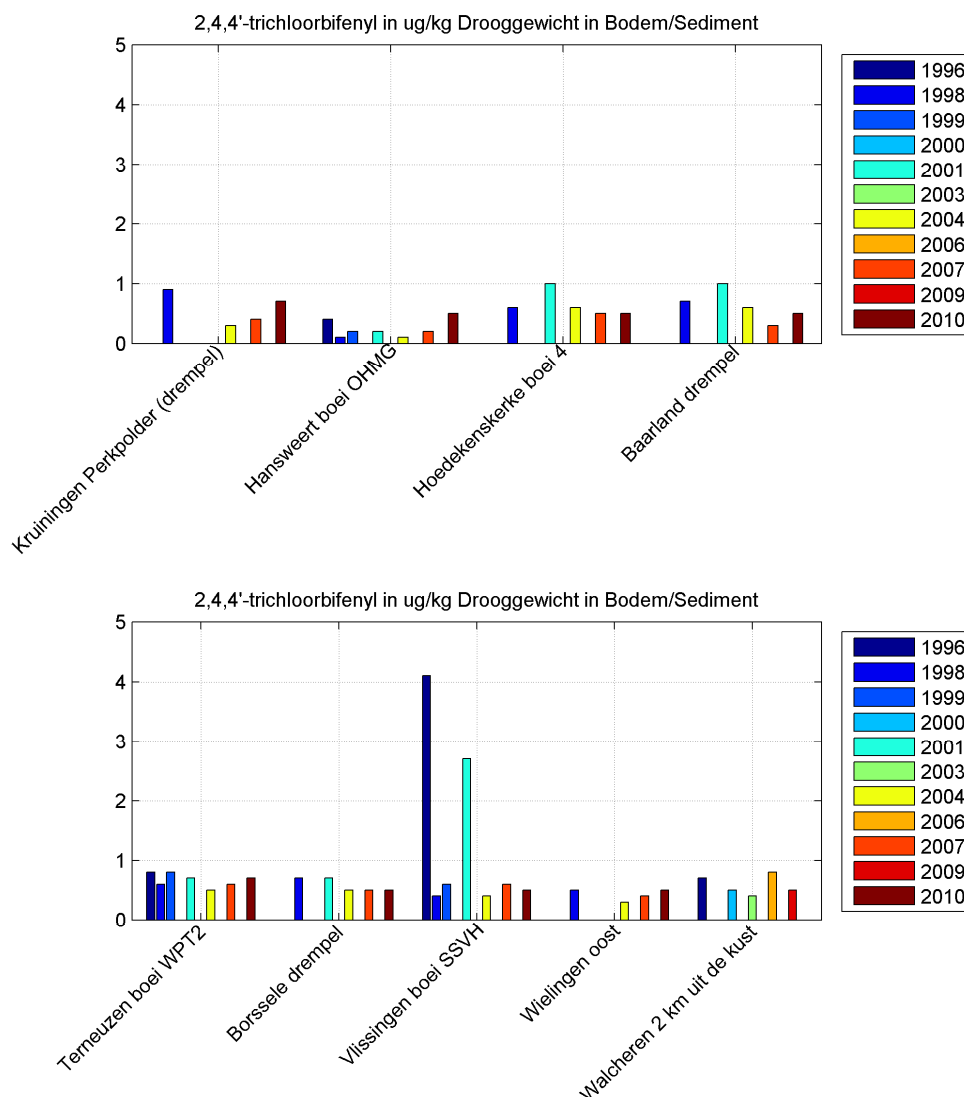
Figuur 3.105 Gemeten gehalten van 2,4,4'-Trichloorbifenyl in bodemsediment van de Westerschelde.
