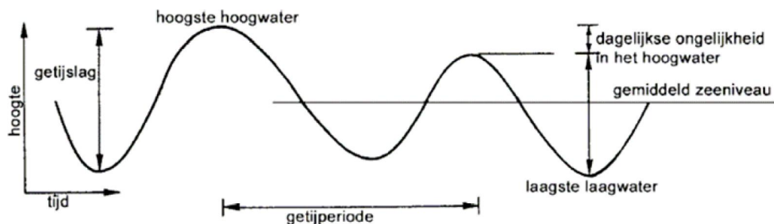
Figuur 2.1 De dagelijkse ongelijkheid in het getij. Opeenvolgende hoog- en laagwaterstanden zijn niet gelijk (naar Van Rijn, 1994)
