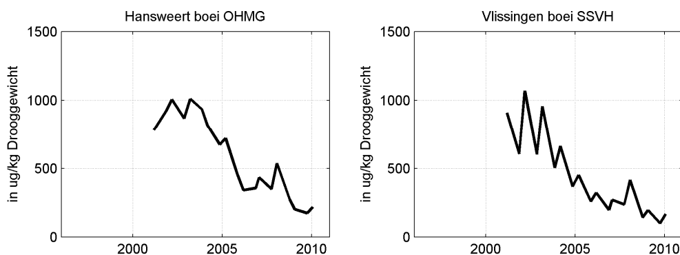
Figuur 3.121 Gemeten gehalten van organotinverbindingen in mosselen ( \mu\text{g/kg} drooggewicht, actieve monitoring) op verschillende stations in de Westerschelde als functie van de tijd.
