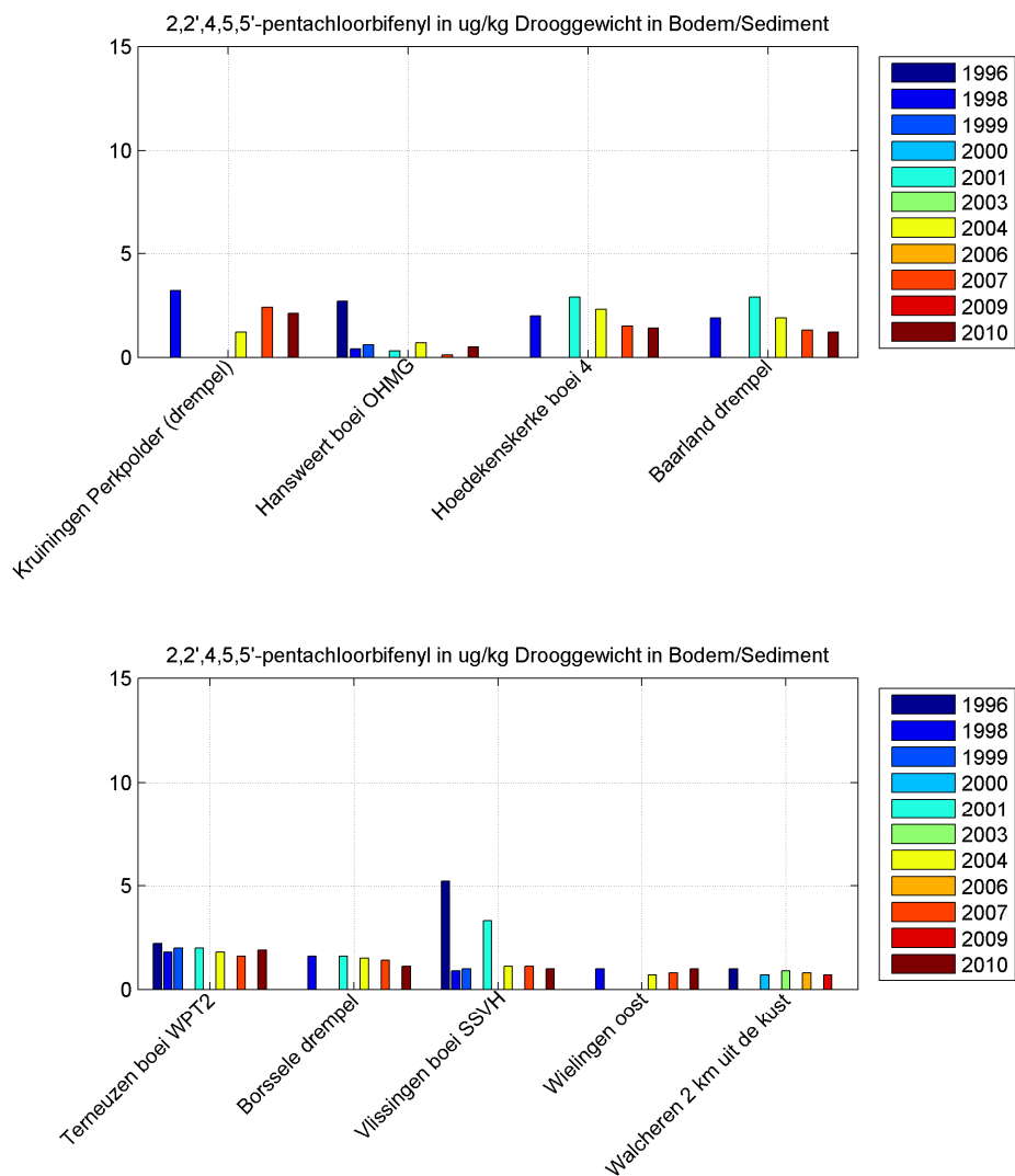
Figuur 3.102 Gemeten gehalten van 2,2',4,5,5'-Pentachloorbifenyyl in bodemsediment van de Westerschelde.
