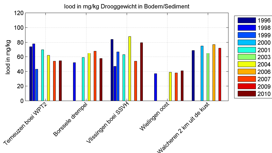
Figuur 3.97 Gemeten gehalten van lood in bodemsediment van de Westerschelde.
