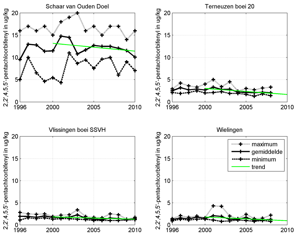
Figuur 3.73 Gemiddelde, minimum- en maximumwaarde per jaar van het gehalte 2,2',4,5,5'-pentachlorobifenyl in zwevende stof op verschillende stations in het estuarium.
