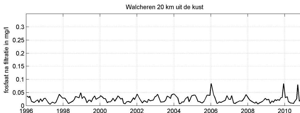
Figuur 3.36 Fosfaat na filtratie in de Westerschelde en de monding
