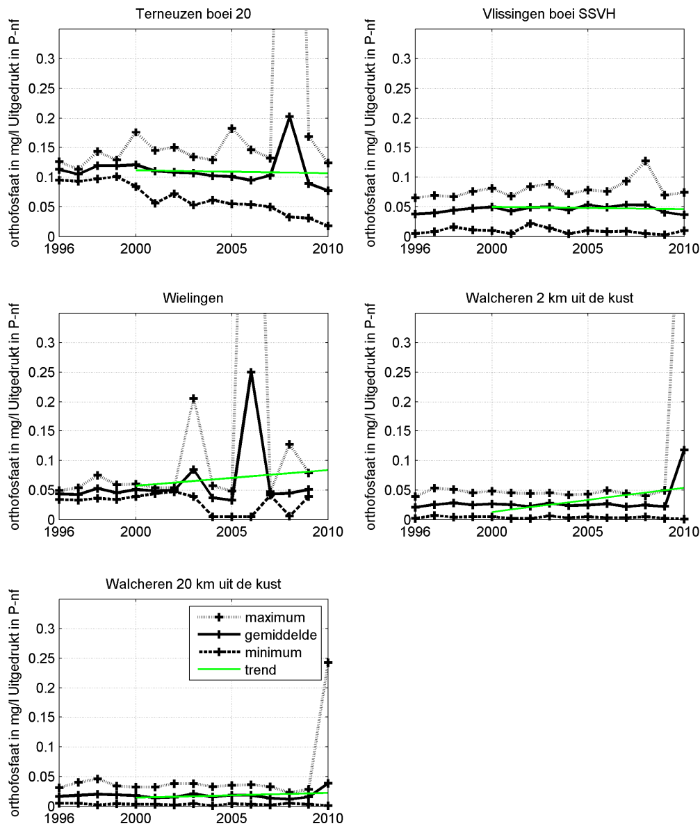
Figuur 3.33 Jaargemiddeld, minimum en maximum orthofosfaat in de Westerschelde en de monding
