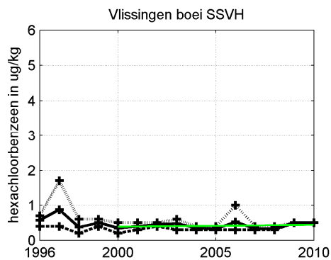
Figuur 3.88 Gemiddelde, minimum- en maximumwaarde per jaar van het gehalte hexachlorobenzene in zwevende stof op verschillende stations in het estuarium.
