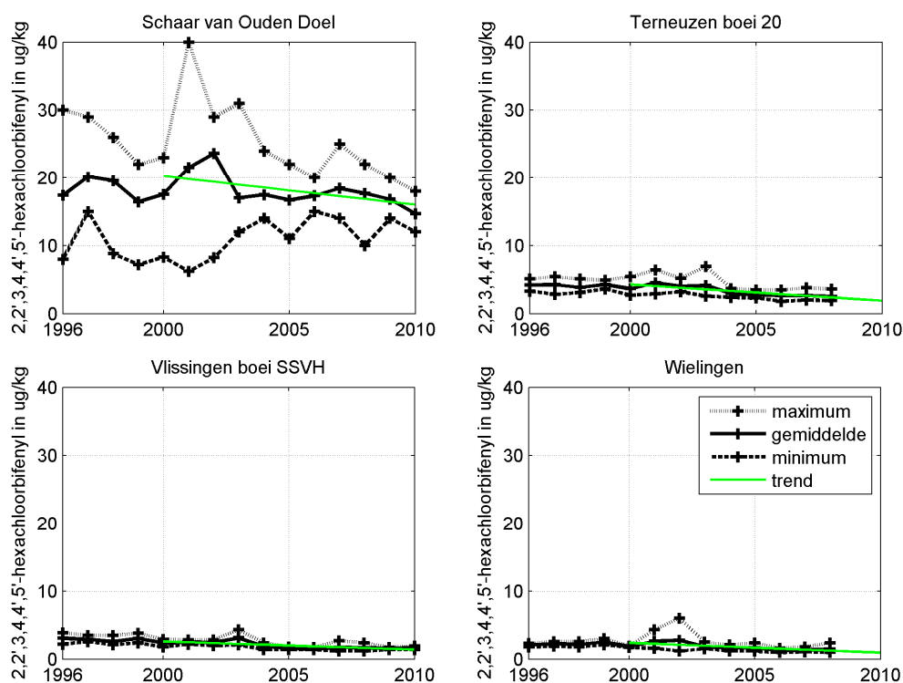
Figuur 3.71 Gemiddelde, minimum- en maximumwaarde per jaar van het gehalte 2,2',3,4,4',5'-hexachlorobifenyl in zwevende stof op verschillende stations in het estuarium.
