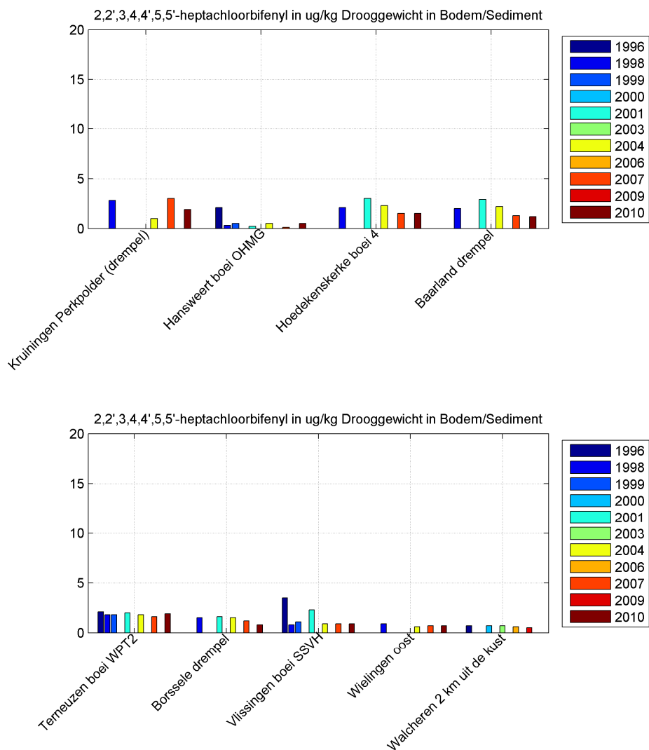
Figuur 3.100 Gemeten gehalten van 2,2',3,4,4',5,5'-Heptachloorbifenyyl in bodemsediment van de Westerschelde.
