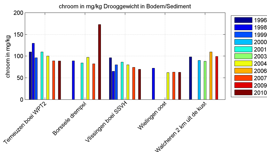
Figuur 3.94 Gemeten gehalten van chromium in bodemsediment van de Westerschelde.
