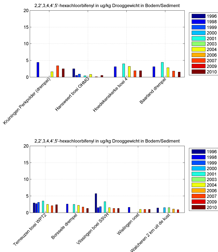
Figuur 3.99 Gemeten gehalten van 2,2',3,4,4',5'-Hexachloorbifenyyl in bodemsediment van de Westerschelde.
