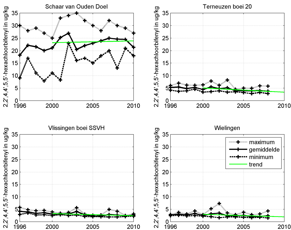
Figuur 3.72 Gemiddelde, minimum- en maximumwaarde per jaar van het gehalte 2,2',4,4',5,5'-hexachlorobifenyl in zwevende stof op verschillende stations in het estuarium.
