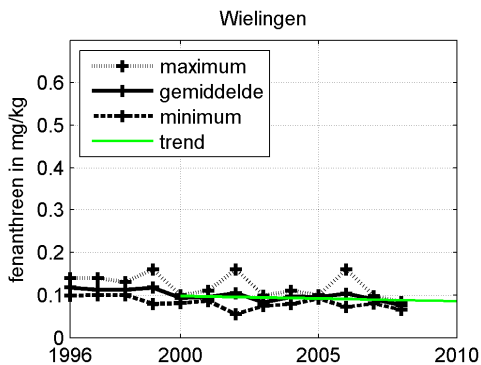
Figuur 3.83 Gemiddelde, minimum- en maximumwaarde per jaar van het gehalte fenantheen in zwevende stof op verschillende stations in het estuarium.
