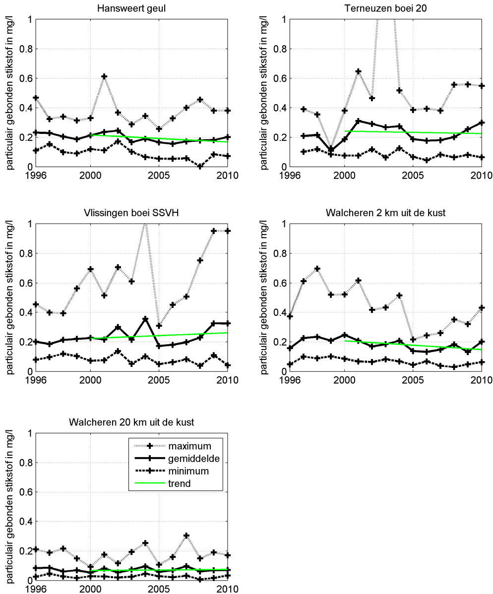
Figuur 3.31 Jaargemiddeld, minimum en maximum particulier gebonden stikstof in de Westerschelde en de monding
