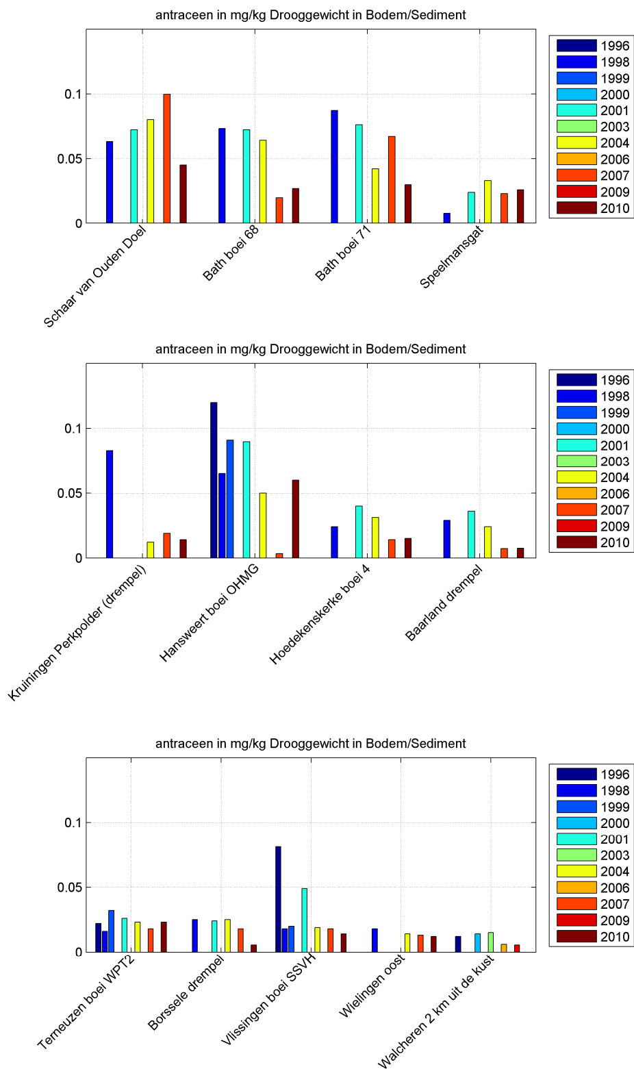
Figuur 3.106 Gemeten gehalten van antracene in bodemsediment van de Westerschelde.
