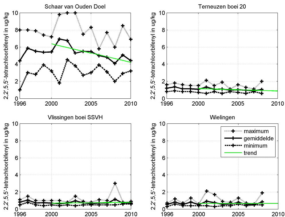
Figuur 3.74 Gemiddelde, minimum- en maximumwaarde per jaar van het gehalte 2,2',5,5'-tetrachloorbifenyl in zwevende stof op verschillende stations in het estuarium.
