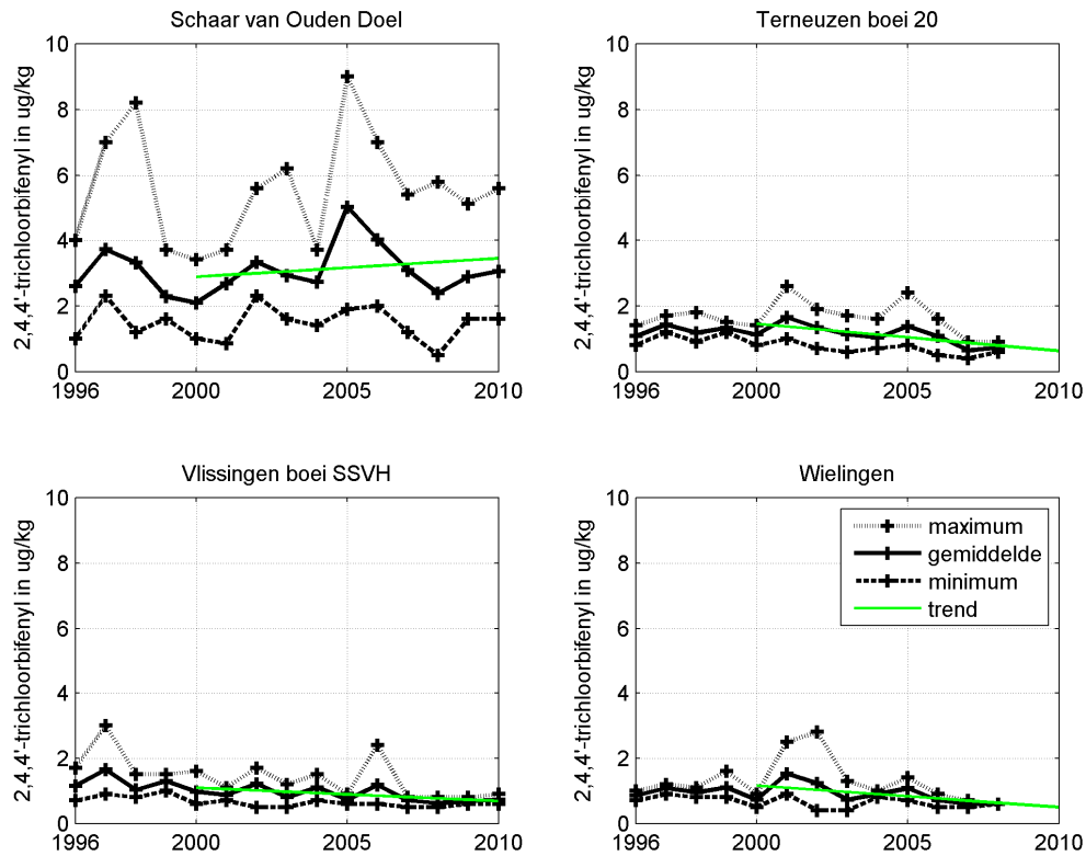
Figuur 3.76 Gemiddelde, minimum- en maximumwaarde per jaar van het gehalte 2,4,4'-trichlorobiphenyl in zwevende stof op verschillende stations in het estuarium.
