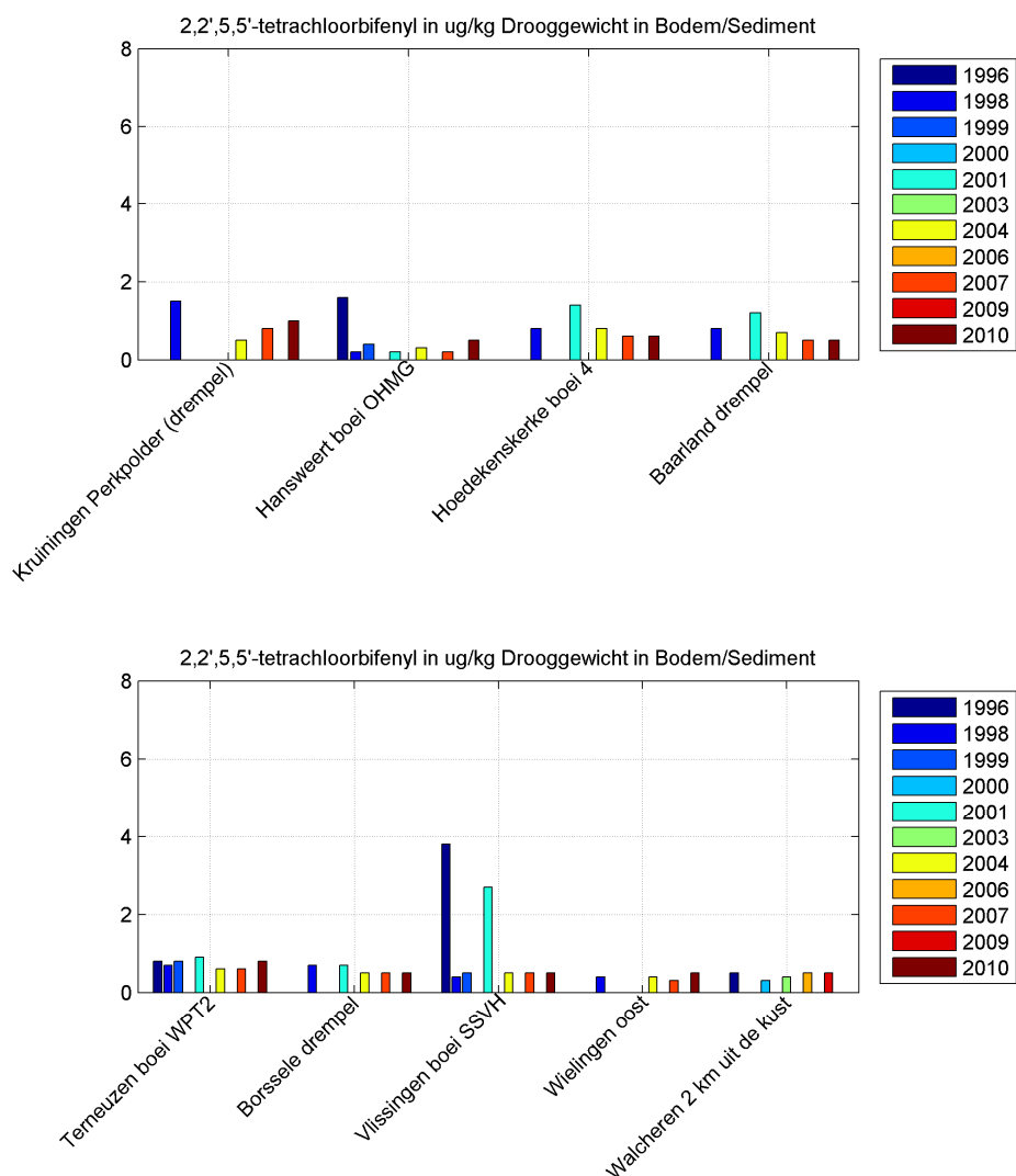
Figuur 3.104 Gemeten gehalten van 2,2',5,5'-Tetrachloorbifenylnyl in bodemsediment van de Westerschelde.
