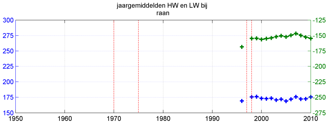
Figuur 2.3 Hoog- en laagwaterstanden op de landelijke en regionale stations. Linker-as (blauw) geeft de hoogwaterstand. Rechter-as (groen) geeft de laagwaterstand
