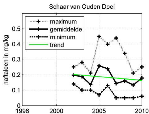
Figuur 3.86 Gemiddelde, minimum- en maximumwaarde per jaar van het gehalte naftaleen in zwevende stof op verschillende stations in het estuarium.
