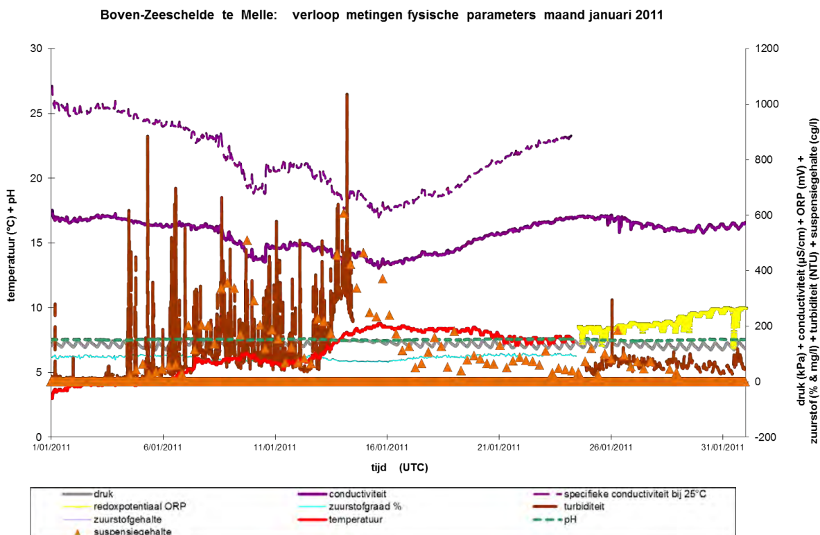
Figuur 130 - Zeeschelde te Melle : verloop van diverse fysische parameters in januari 2011, waarin de wasperiode van half januari 2011 te zien is
