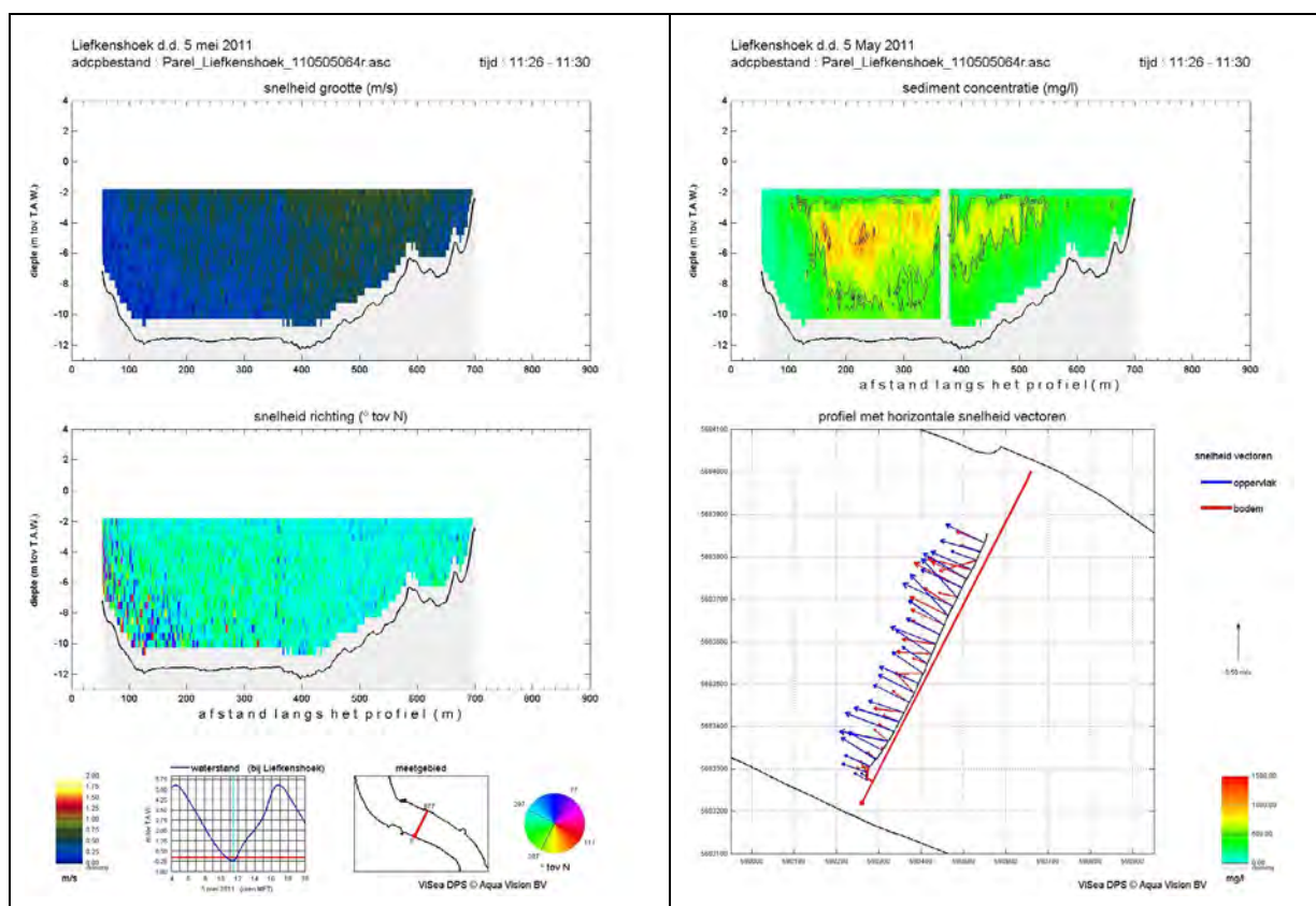
fig. 186 - Beneden-Zeeschelde te Liefkenshoek - ADCP-meting 5 mei 2011 - meetresultaten stroming en suspensiegehalte bij LW
