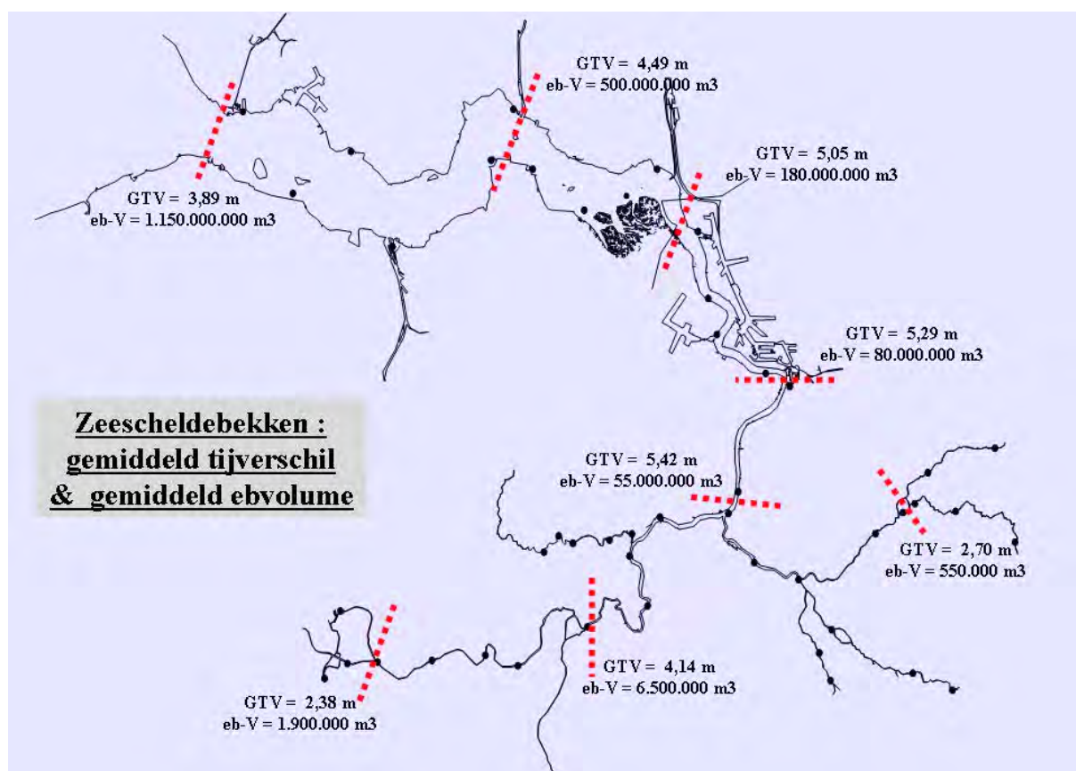
Figuur 5 - Zeescheldebekken: algemeen liggingsplan met aanduiding van gemiddelde tijverschillen (GTV) (in m) en gemiddelde eb-volumes (eb-V) (in m³) op enkele kenmerkende locaties
