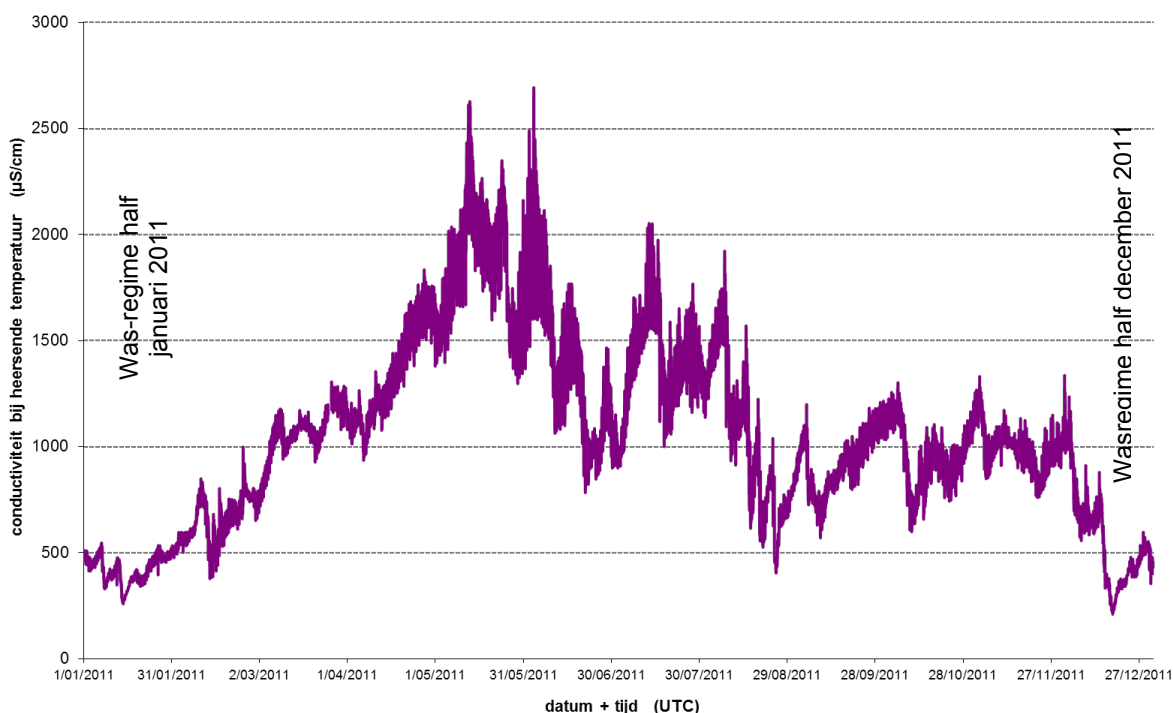
Figuur 163 - Beneden-Nete te Duffelsluis : jaarverloop 2011 van de conductiviteit bij heersende temperatuur
