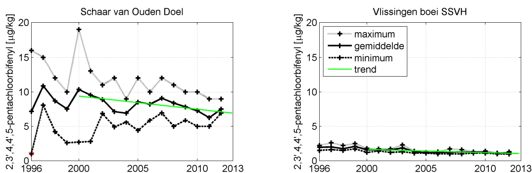
Figuur 4.18 Jaargemiddelde, jaarminimum en jaarmaximum van het gehalte 2,3',4,4',5-pentachloorbifenyyl (PCB118) in zwevende stof
