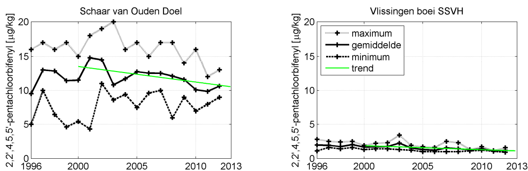
Figuur 4.16 Jaargemiddelde, jaarminimum en jaarmaximum van het gehalte 2,2',4,4',5,5'-pentachloorbifenyyl (PCB101) in zwevende stof
