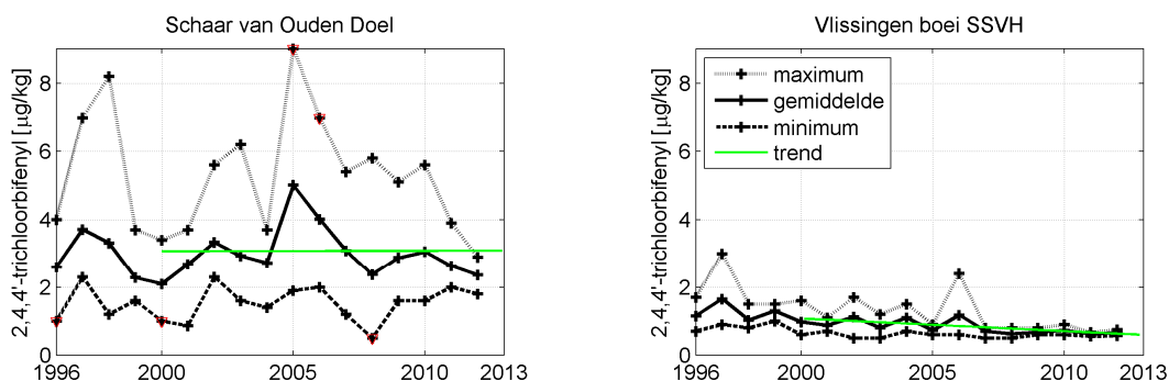
Figuur 4.19 Jaargemiddelde, jaarminimum en jaarmaximum van het gehalte 2,4,4'-trichlorobifenyl (PCB28) in zwevende stof
