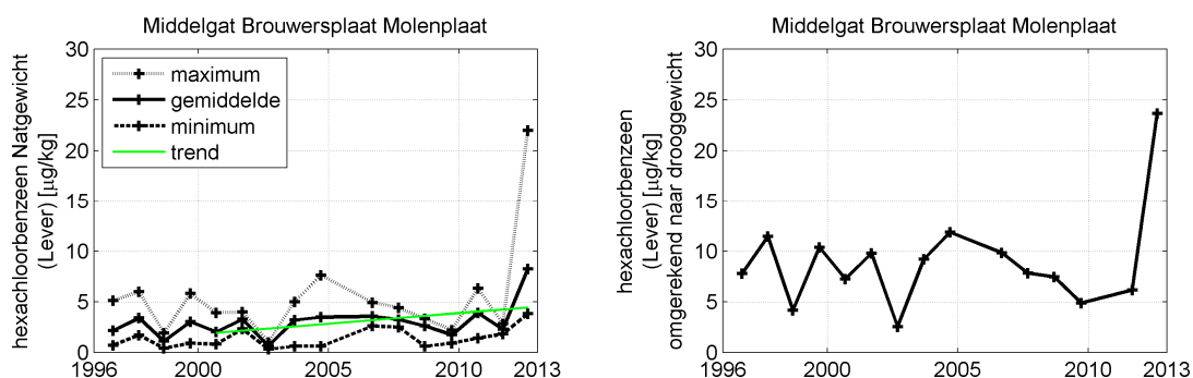
Figuur 5.6 Hexachlorobenzene in bot op locatie Middelgat, Brouwersplaat, Molenplaat in de Westerschelde
