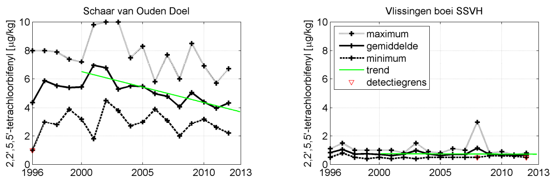
Figuur 4.17 Jaargemiddelde, jaarminimum en jaarmaximum van het gehalte 2,2',5,5'-tetrachloorbifenyyl (PCB52) in zwevende stof
