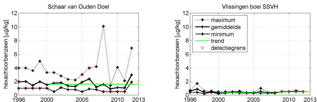
Figuur 4.31 Jaargemiddelde, jaarminimum en jaarmaximum van het gehalte hexachloorbenzeen (HCB) in zwevende stof
