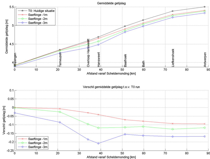
Figuur 4.13: Berekende veranderingen van de getijslag met Finel2D na bodemverlagingen van 1, 2 en 3 m van het Land van Saeftinge (pers. comm. Gerard Dam).
