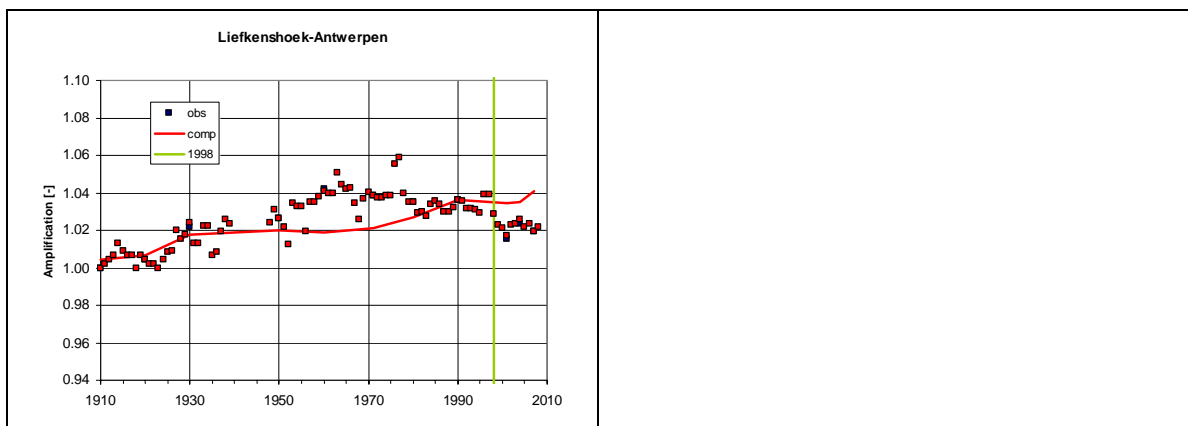
Figuur 3.19: Verloop van de amplificatie tussen Liefkenshoek en Antwerpen voor alle jaren.
