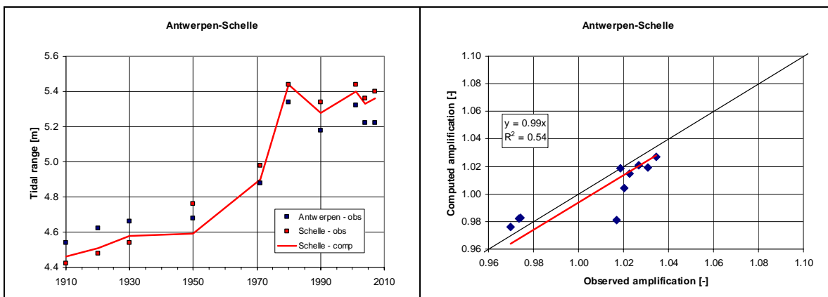
Figuur 3.22: Antwerpen-Schelle: getijslag (links) en correlatie waargenomen en berekende amplificatie (rechts).
