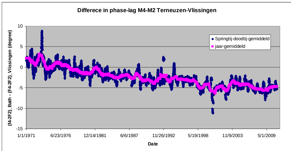
Figuur 3.15 Verschil in relatief faseverschil tussen viermaaldaagse en dubbeldaagse getij tussen Terneuzen en Vlissingen.
